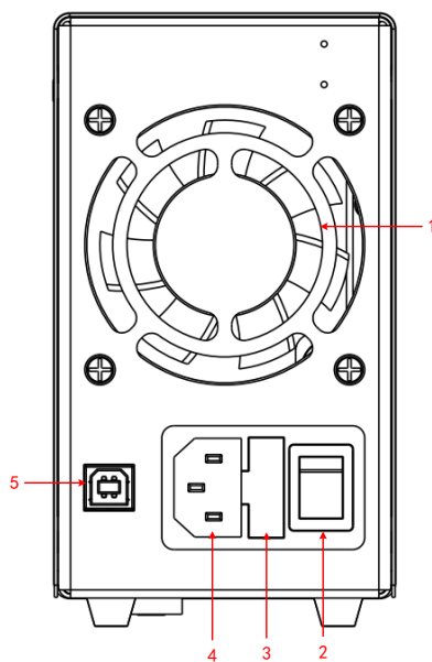
图 2-2 后面板概览
