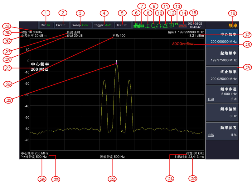
图 3-7 用户界面
