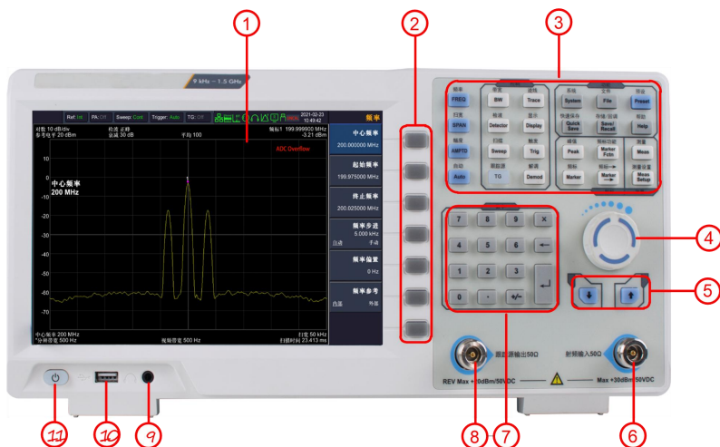
图 4-1 前面板概览
