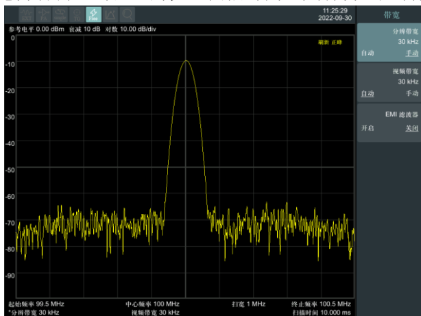
图 3-9 设置扫宽
