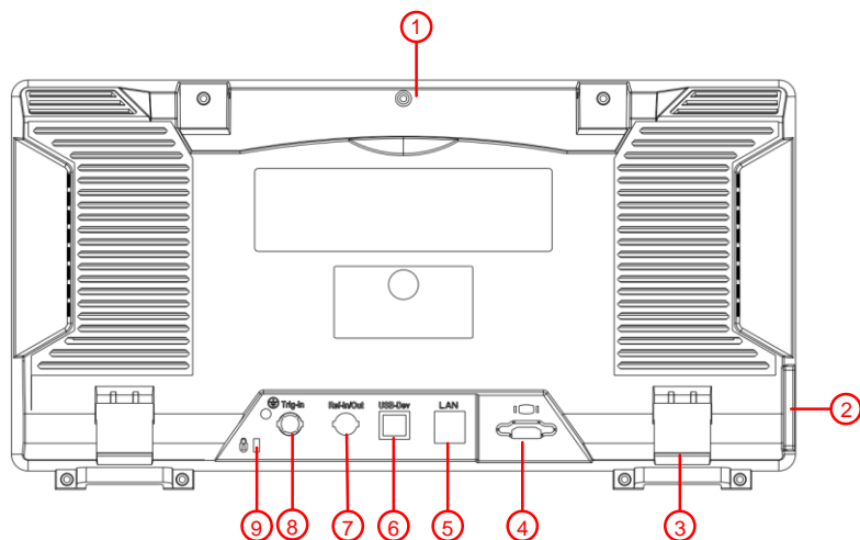
图 3-6 后面板视图
