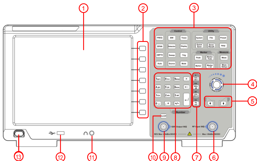
图 3-1 前面板概览
