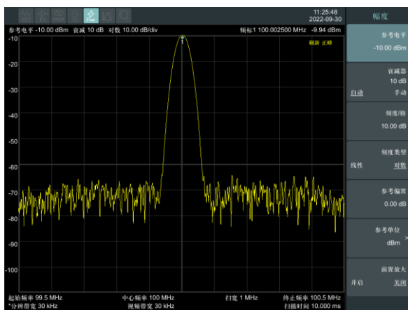
图 3-10 设置参考电平
