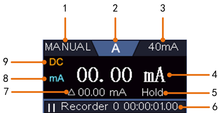
图 5-3：万用表显示窗
