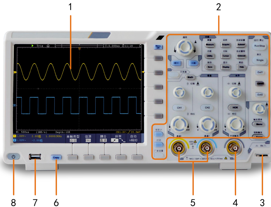
图 3-1: 示波器前面板
