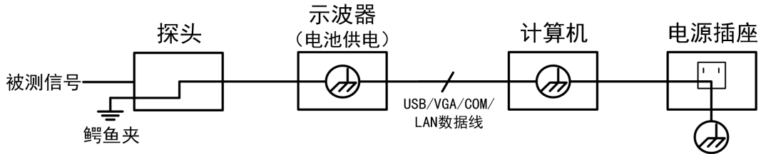
示波器通过端口与计算机（交流供电）连接时的内部地线连接示意图：
