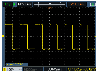
图 3-4：自动设置
