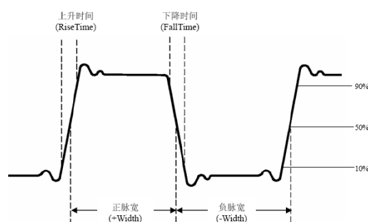
图 3-10：时间参数定义示意
