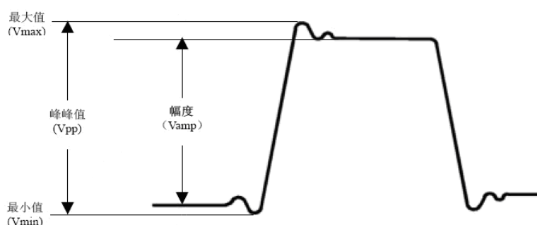
图 3-9：电压参数定义示意（顶端平整有脉冲信号）
