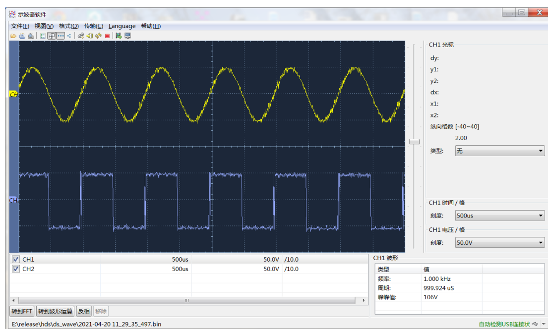
图 6-1: 通过 USB 接口与计算机连接
