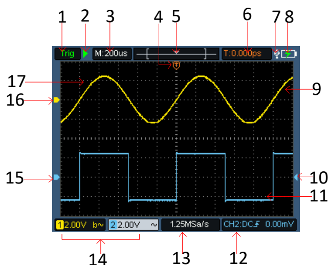
图 3-3：示波器界面
