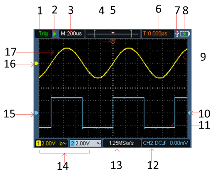
图 3-3：示波器界面
