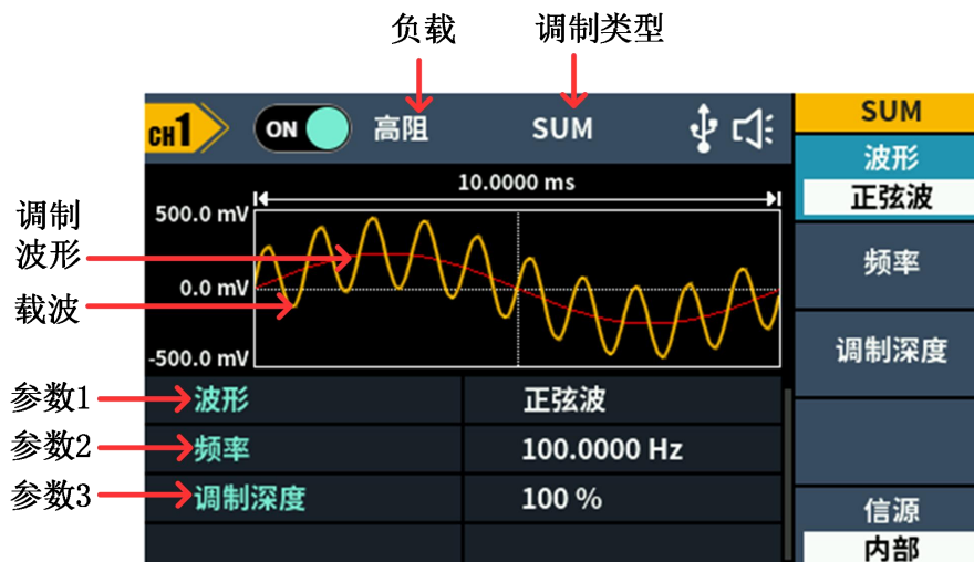
图 5-27 总和调制的用户界面
