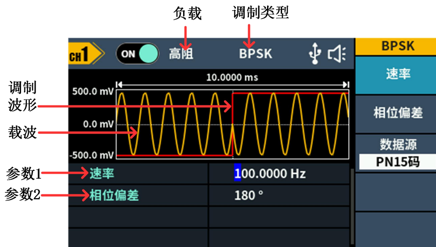
图 5-24 二相相移键控调制的用户界面
