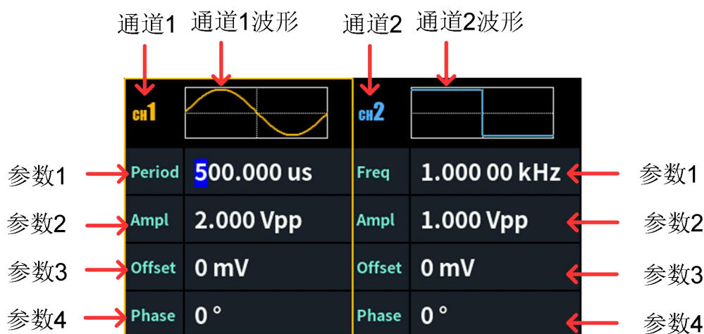
图 5-1: 双通道显示 (Both) 界面
