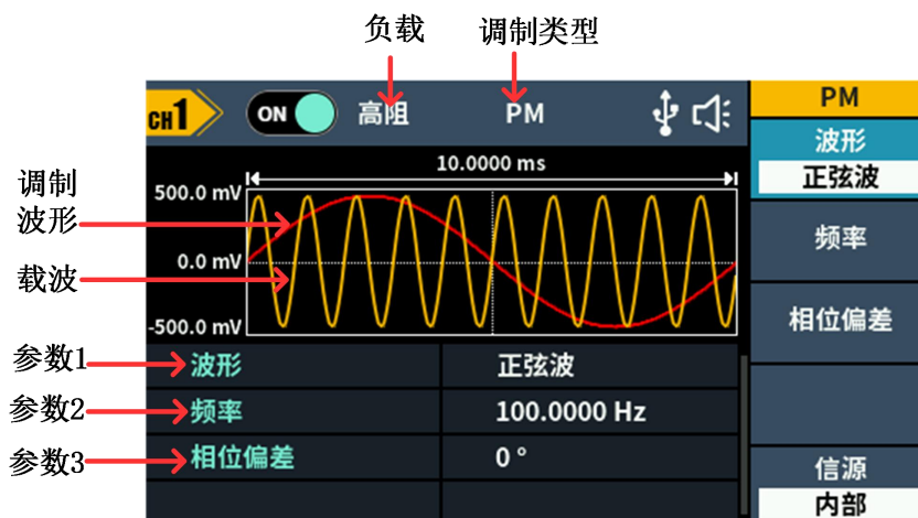
图 5-17：相位调制的用户界面
