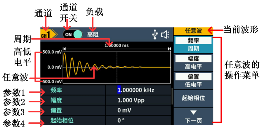
图 5-10: 任意波用户界面
