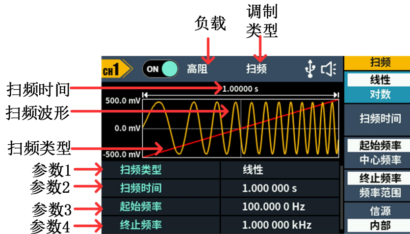
图 5-11: 扫频模式的用户界面
