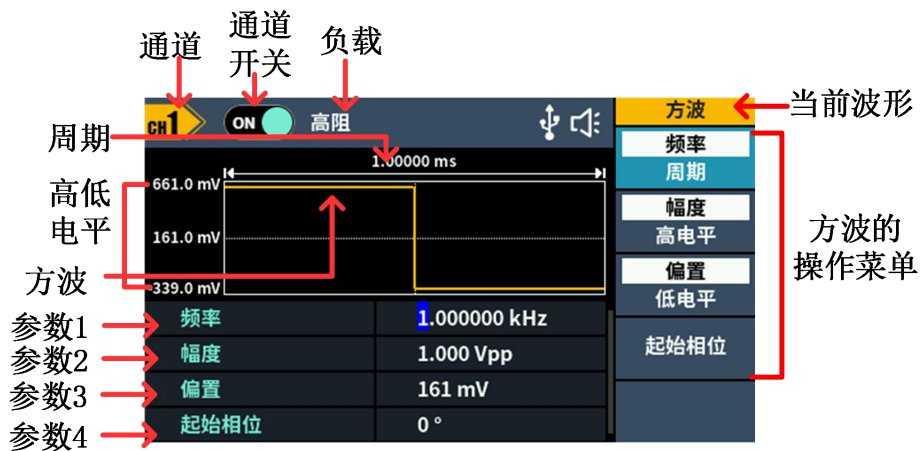
图 5-4：方波用户界面
