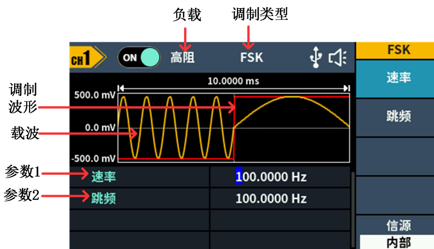
图 5-21: 频移键控调制的用户界面
