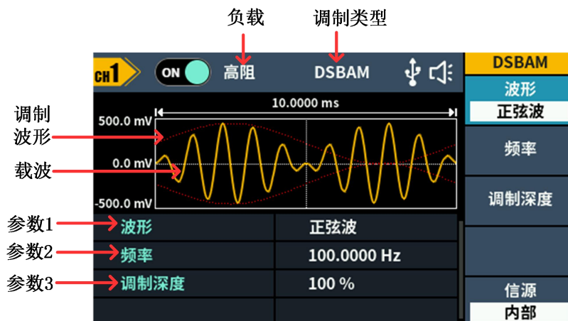
图 5-15: 双边振幅调制的用户界面
