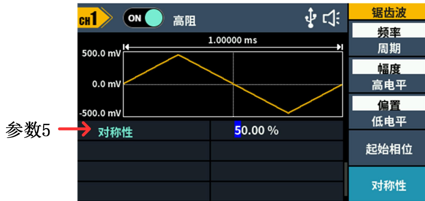
图 5-5: 锯齿波用户界面
