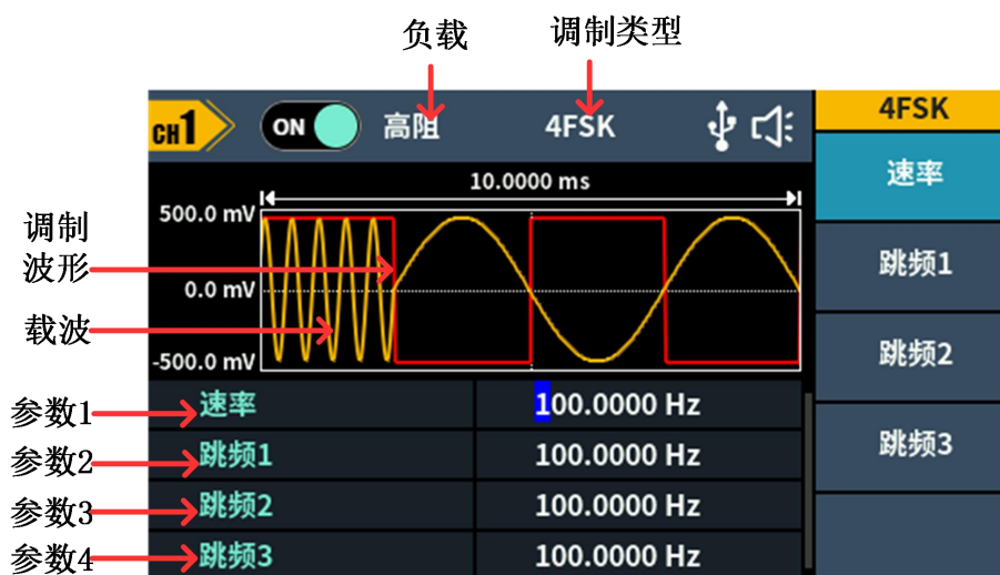
图 5-23 四进制频移键控调制的用户界面
