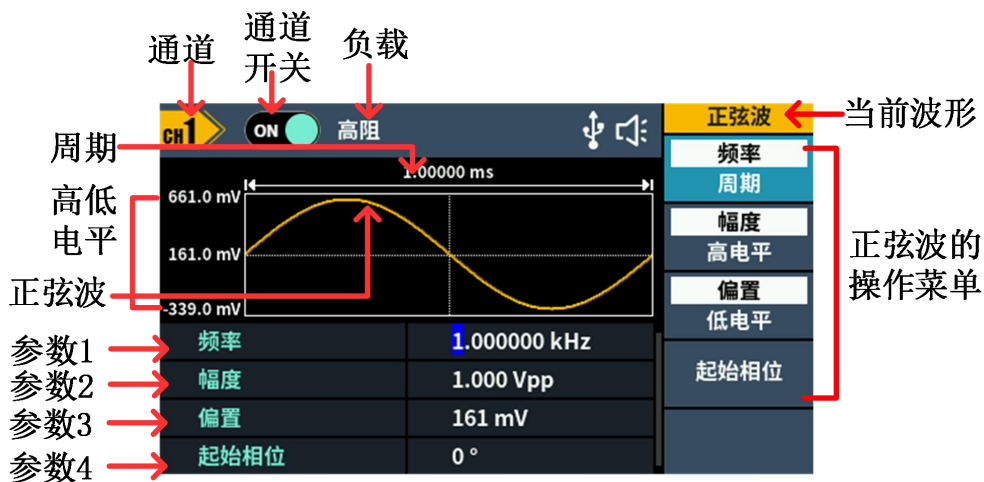
图 5-2：正弦波用户界面
