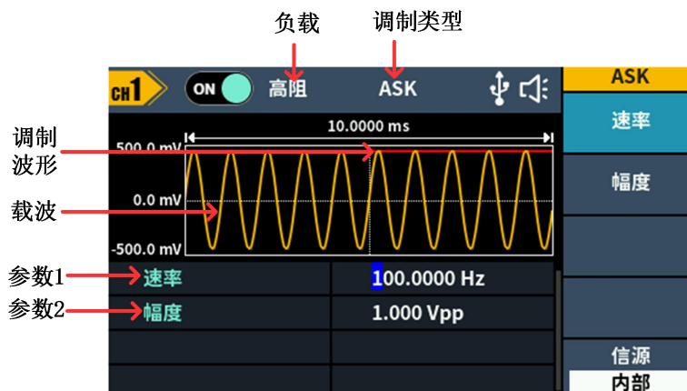
图 5-19 幅移键控调制的用户界面
