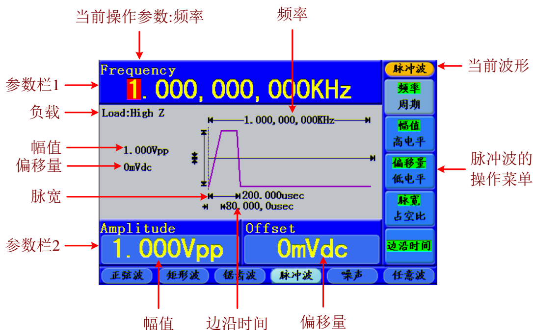
图 5-7：脉冲波用户界面
