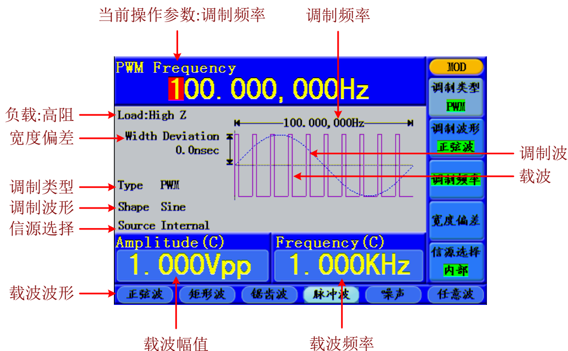
图 5-16：脉宽调制的用户界面
