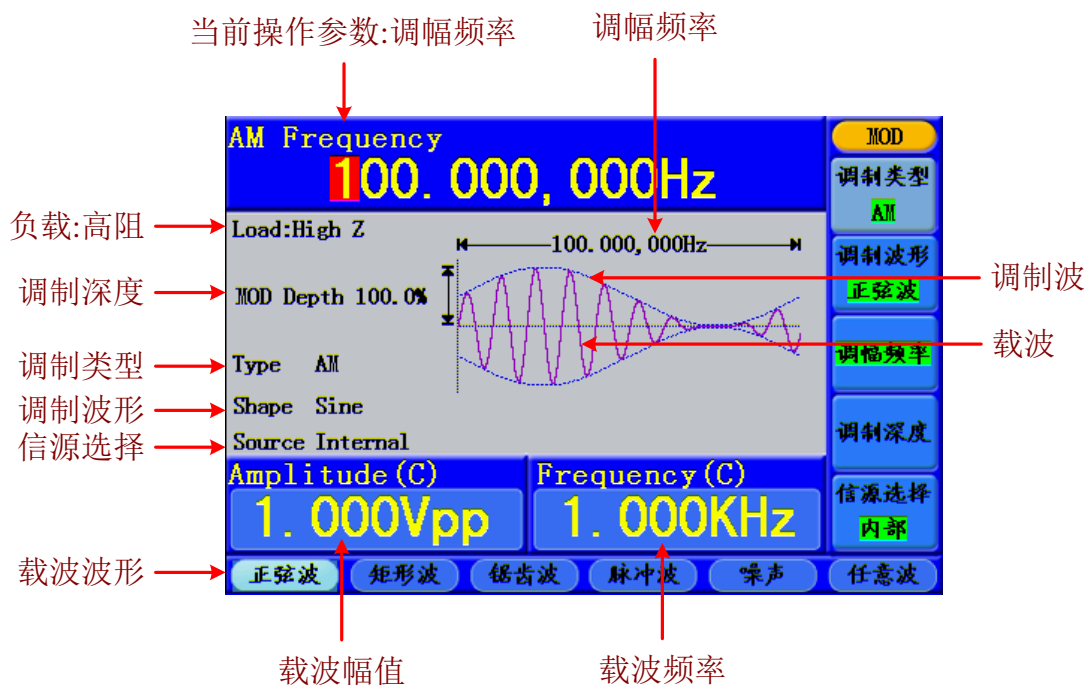
图 5-12: 振幅调制的用户界面
