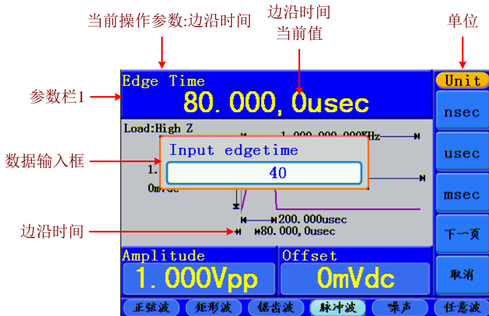
图 5-9：设置脉冲波的边沿时间
