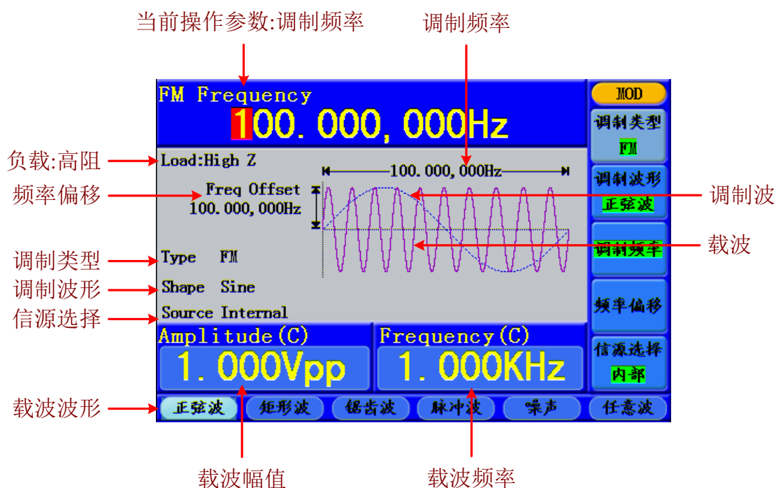
图 5-13：频率调制的用户界面
