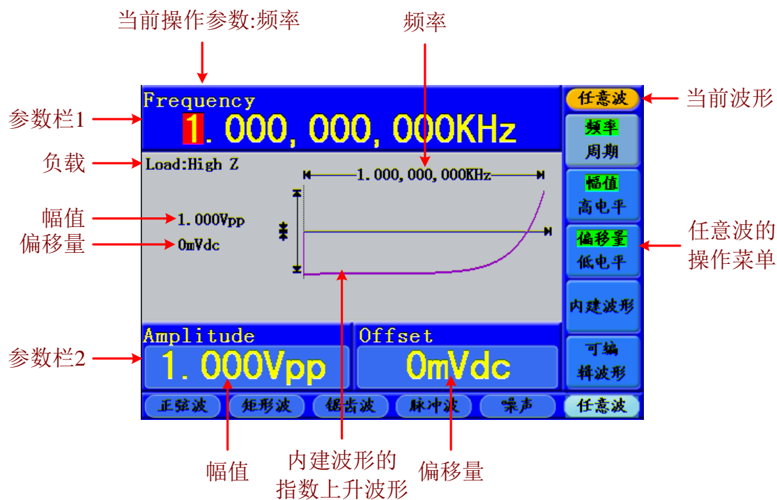
图 5-11：任意波用户界面
