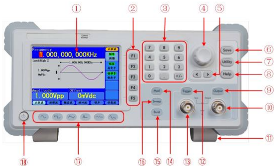
图 4-1 前面板概览
