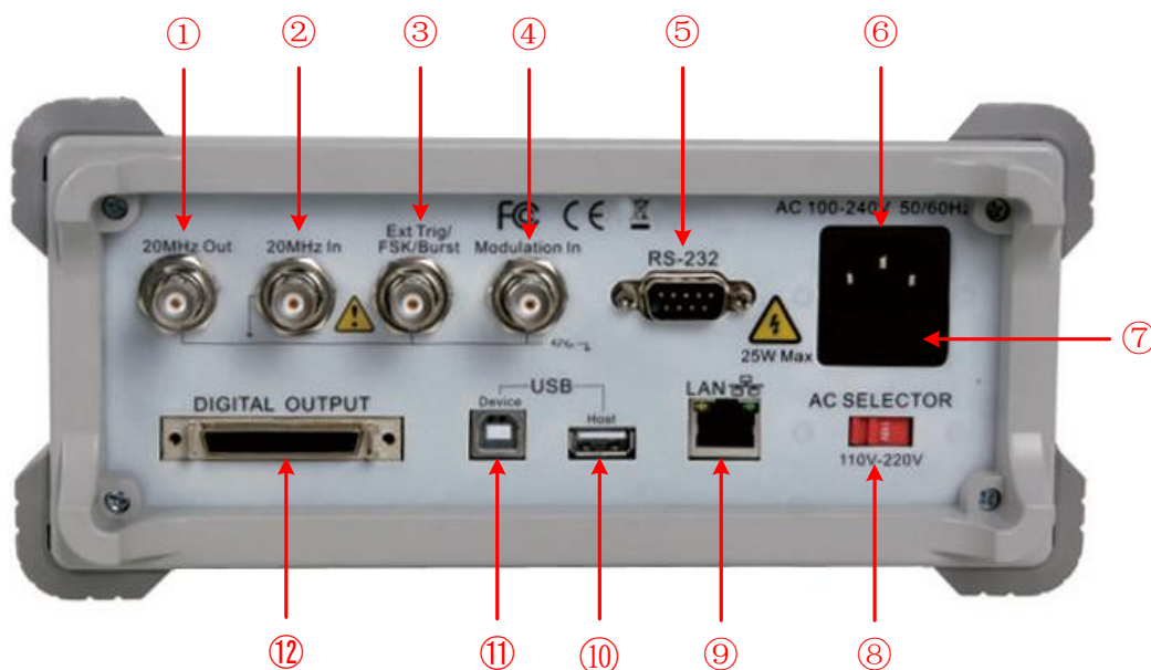
图 4-2 后面板概览
