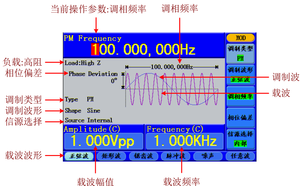
图 5-14：相位调制的用户界面
