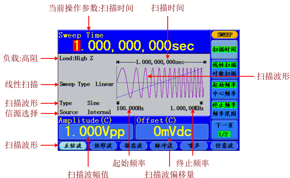
图 5-17：扫描模式的用户界面
