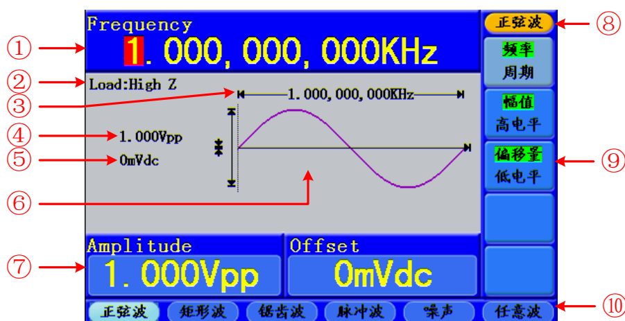
图 4-3 用户界面（以正弦波为例）
