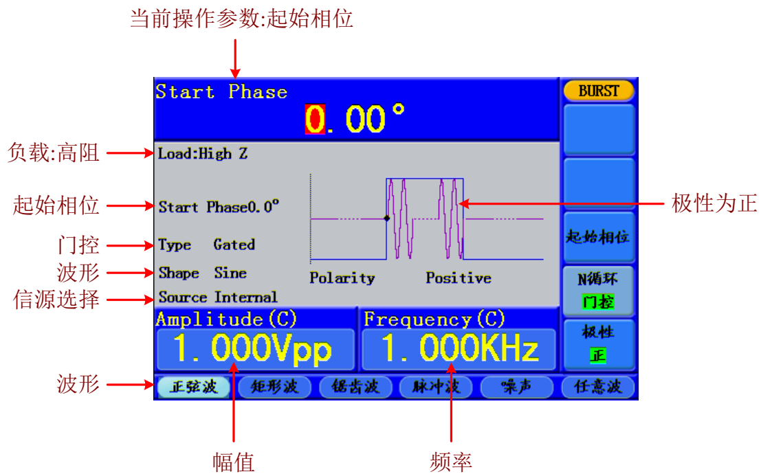
图 5-19: 门控脉冲串的用户界面
