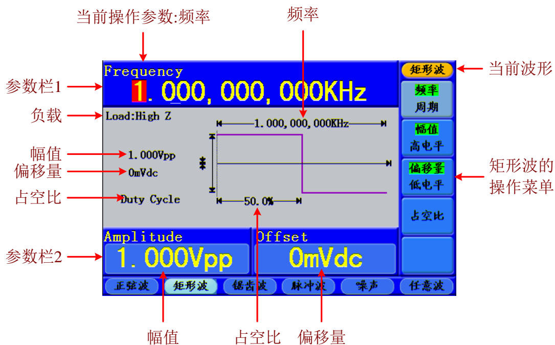
图 5-3：矩形波用户界面
