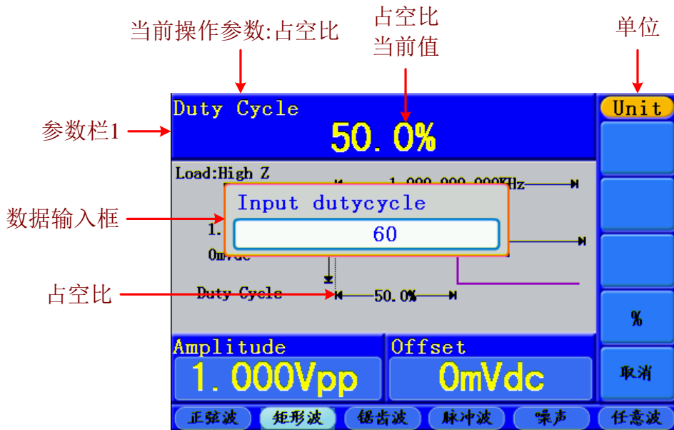
图 5-4：设置矩形波的占空比
