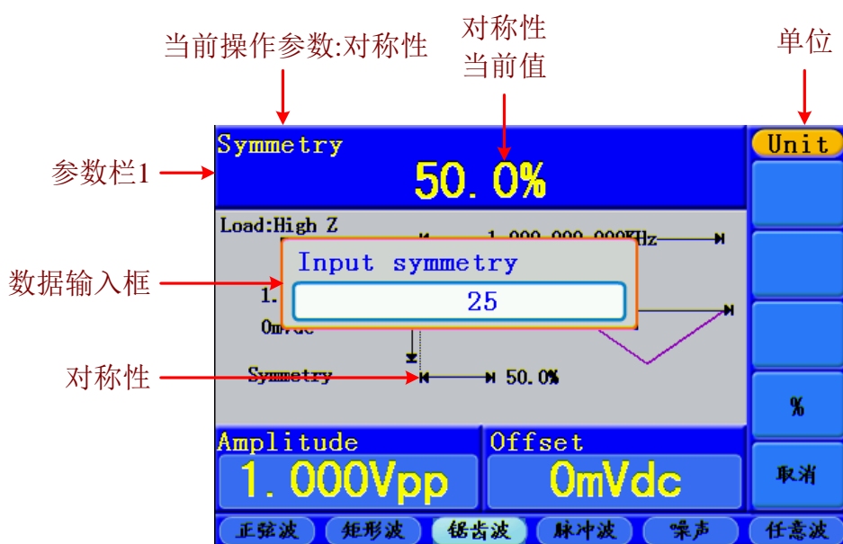
图 5-6: 设置锯齿波的对称性
