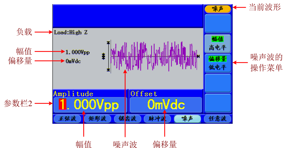
图 5-10: 噪声波用户界面
