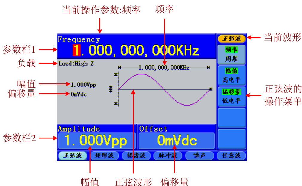
图 5-1：正弦波用户界面
