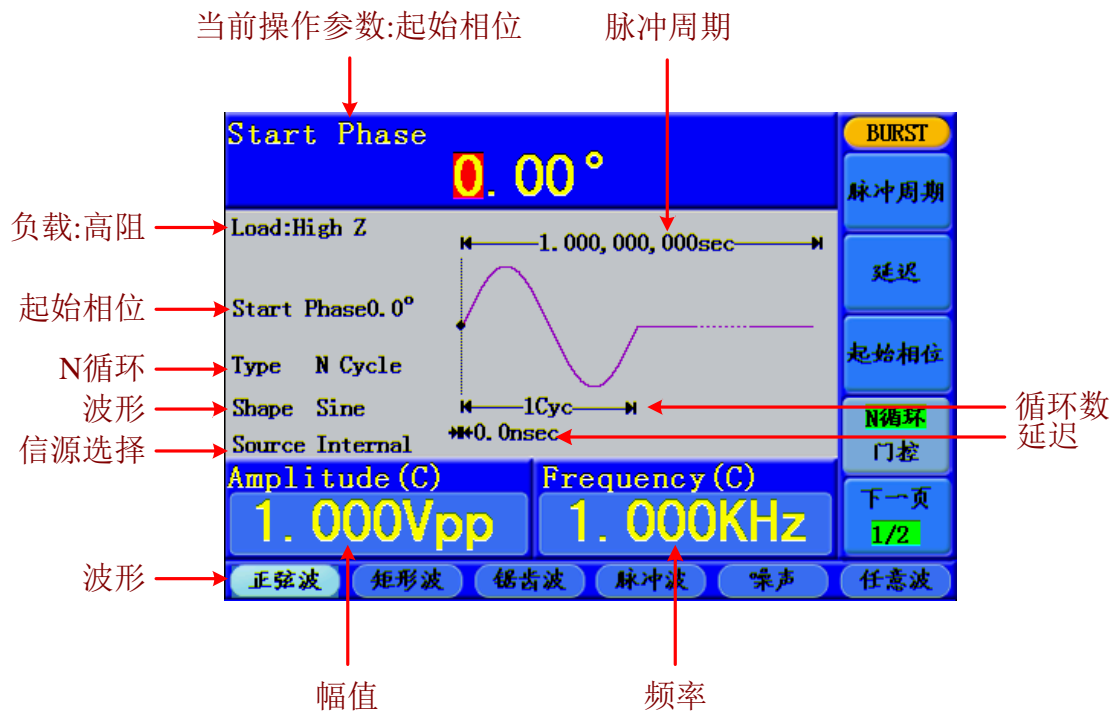
图 5-18: N 循环脉冲串的用户界面
