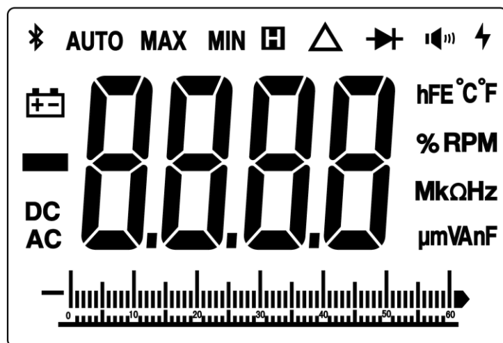
图 2-2 显示屏
