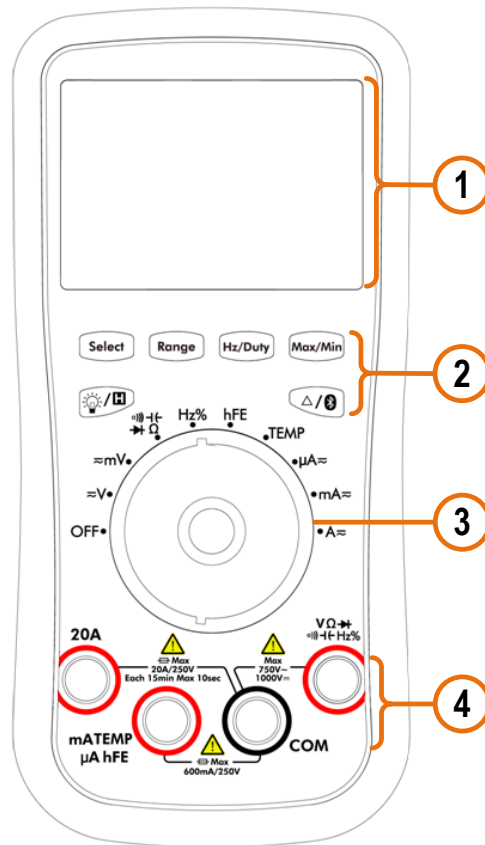
图 2-1 前面板概览（以 B35 为例）
