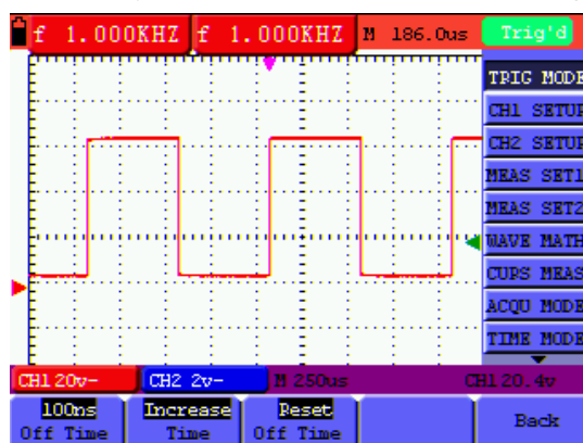
figure45:Trigger Holdoff
